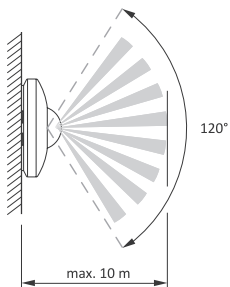
Montaż naścienny
